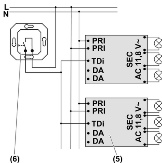
Afbeelding 5: Aansluitschema met installatiedrukknop
